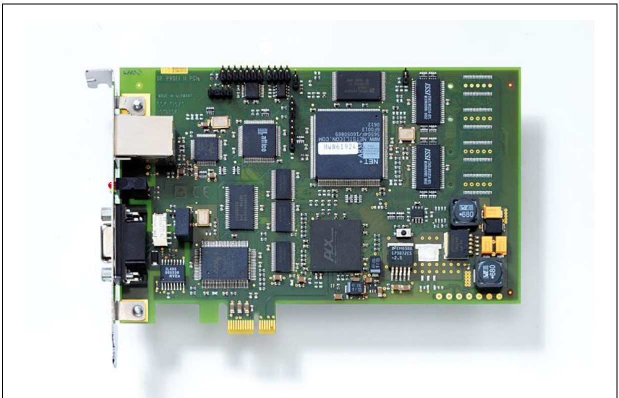
Abbildung 1: DF PROFI II PCIe – Baugruppe
